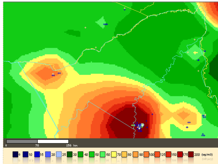
DISTRIBUCIÓN DEL MONÓXIDO DE CARBONO EN LA REGIÓN DE FECHA 12-AGO-2010
