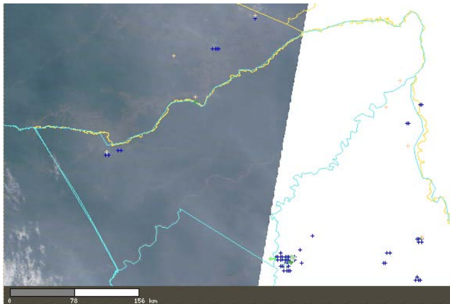
DISTRIBUCIÓN DE FOCOS DE CALOR DEL DEPARTAMENTO CON IMAGEN MODIS DE FECHA 12-AGO-2010
